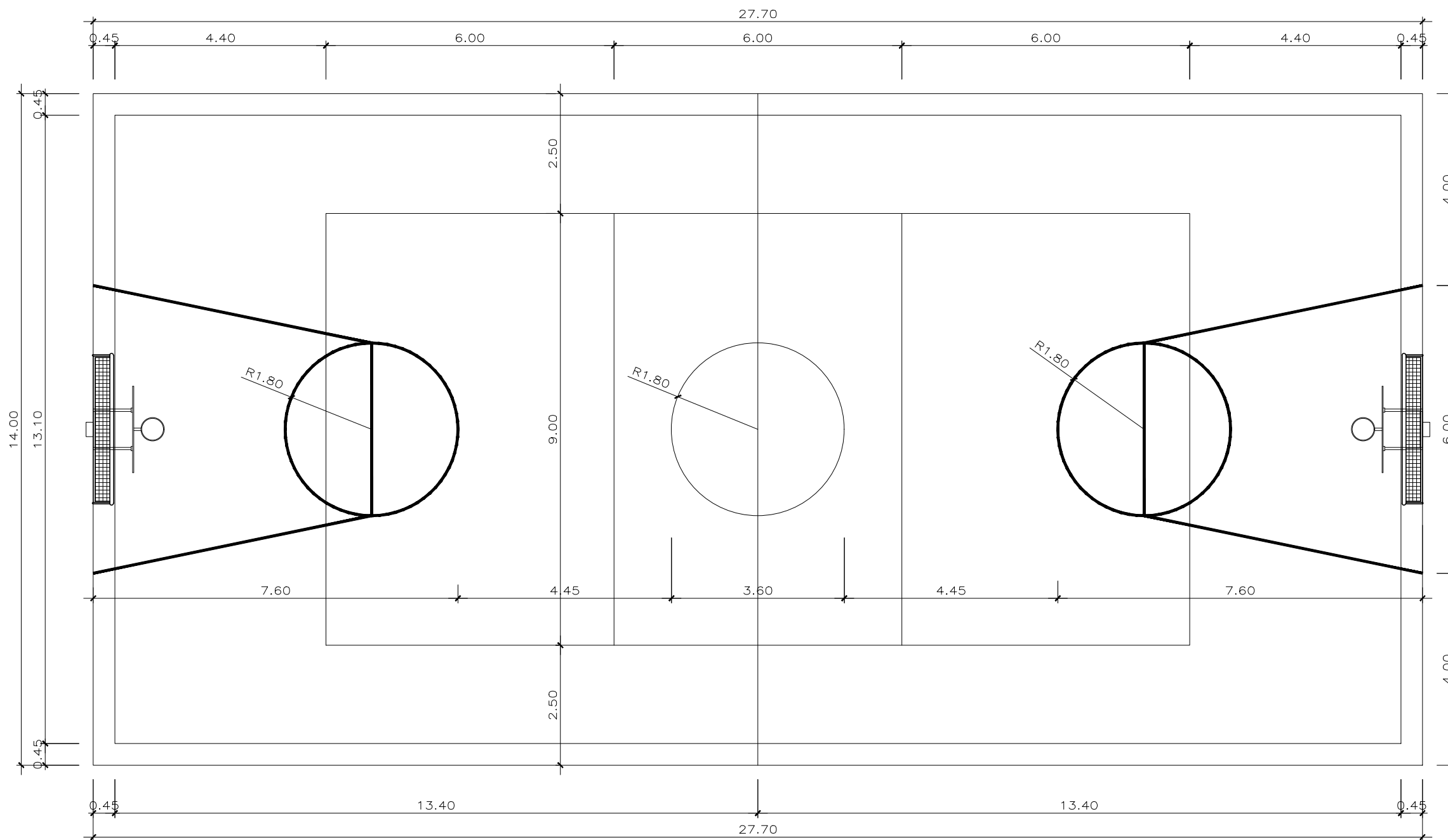
PLANTA BAIXA - QUADRA DE ESPORTES ESCALA 1:100
