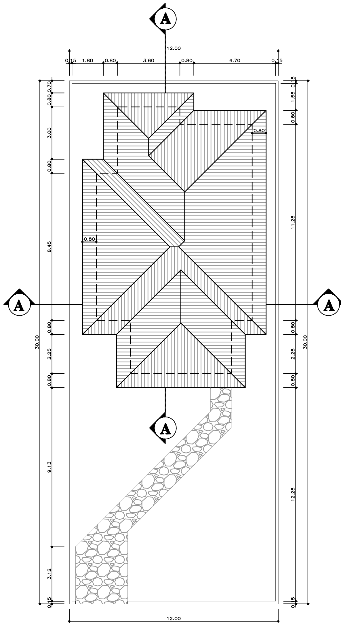
PLANTA DE LOCAÇÃO E COBERTURA ESCALA 1:125
