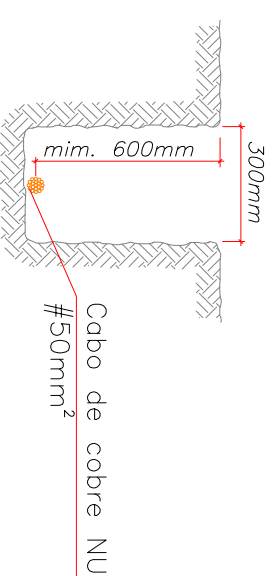
DETALHE "E" DIMENSÃO DA VALA PARA MALHA DE TERRA S/ ESCALA
