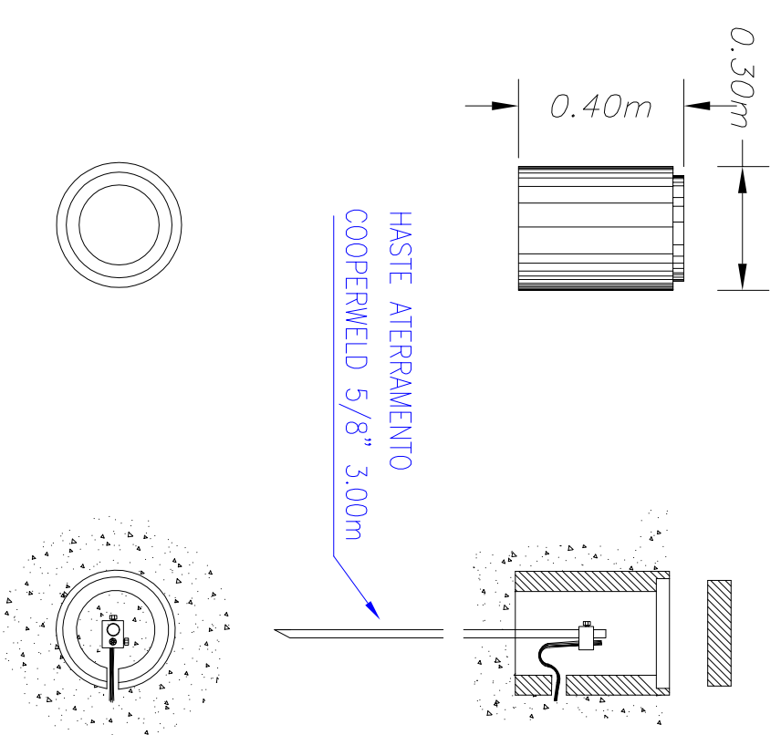
DETALHE "G" CAIXA CONCRETO PARA INSPEÇÃO DE ATERRAMENTO S/ ESCALA
