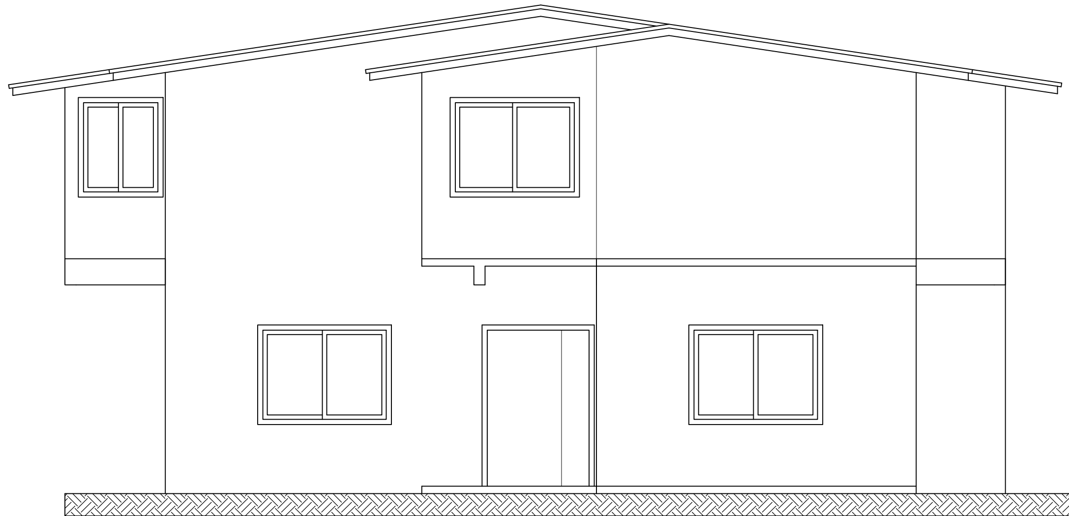
ELEVAÇÃO FRONTAL ESCALA 1:50
