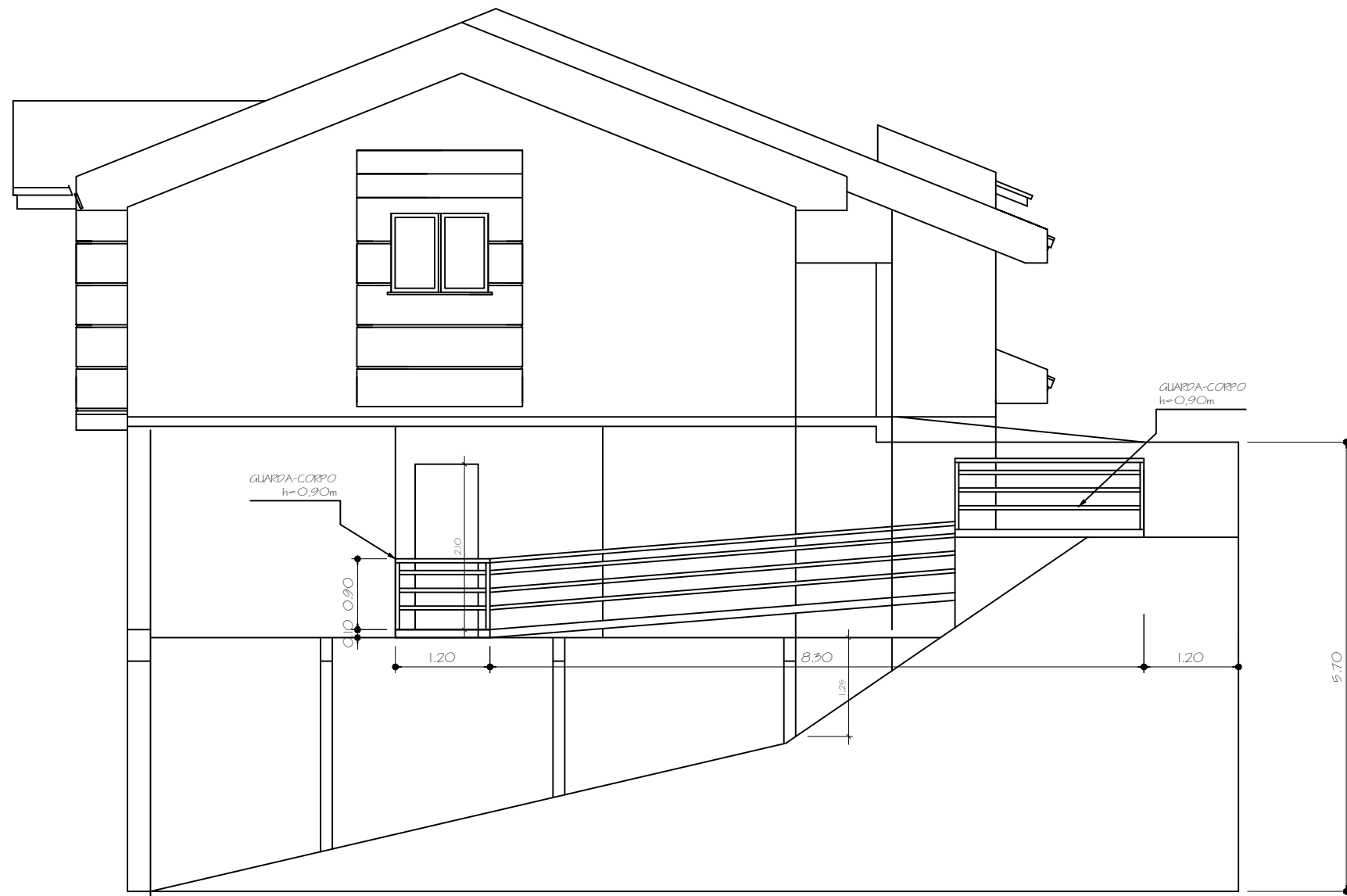
ELEVAÇÃO LATERAL ESQUERDA - RAMPA ESCALA 1:50
