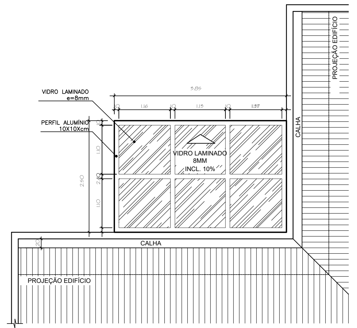
PLANTA BAIXA - PERGOLADO FUNDOS ESCALA 1:50
