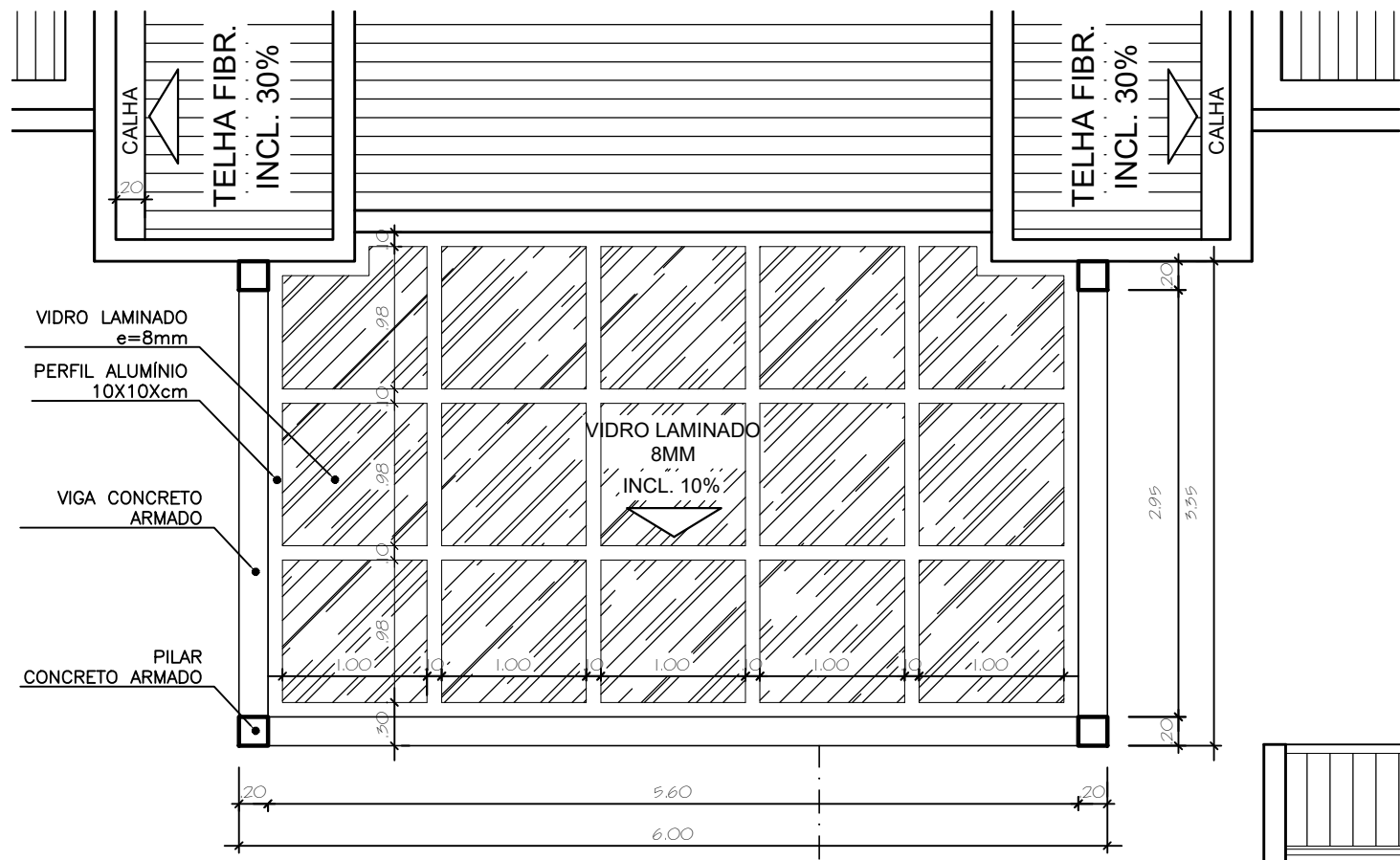
PLANTA BAIXA - PERGOLADO FRONTAL ESCALA 1:50
