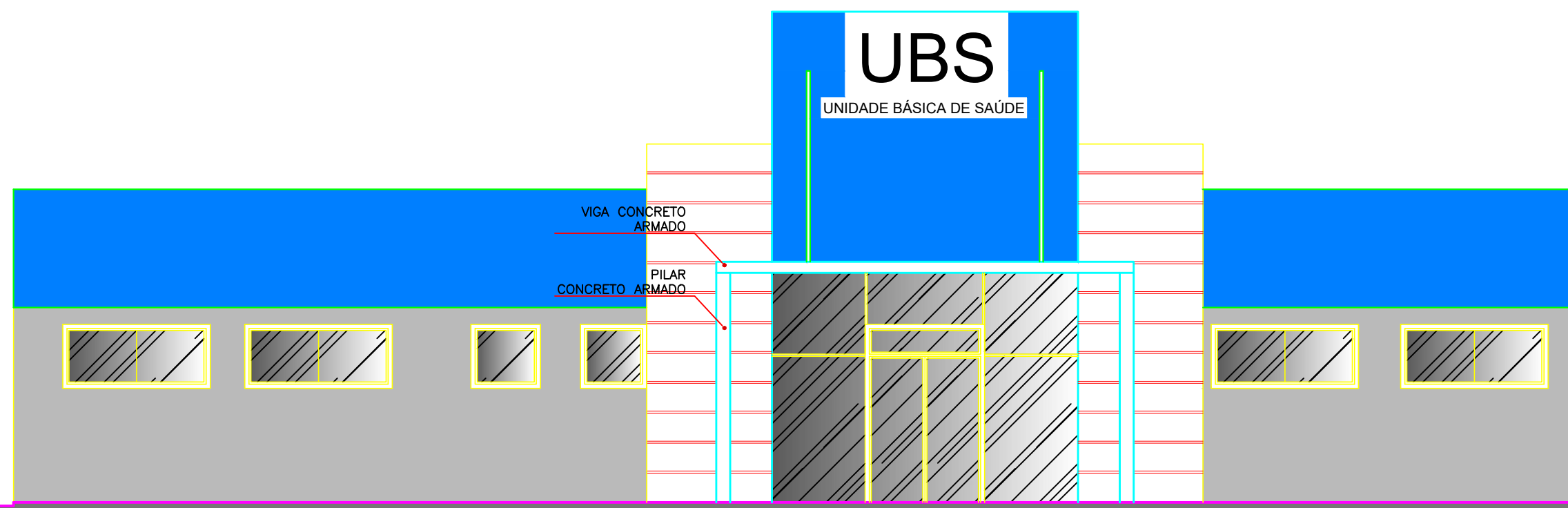
ELEVAÇÃO FRONTAL ESCALA 1:75
