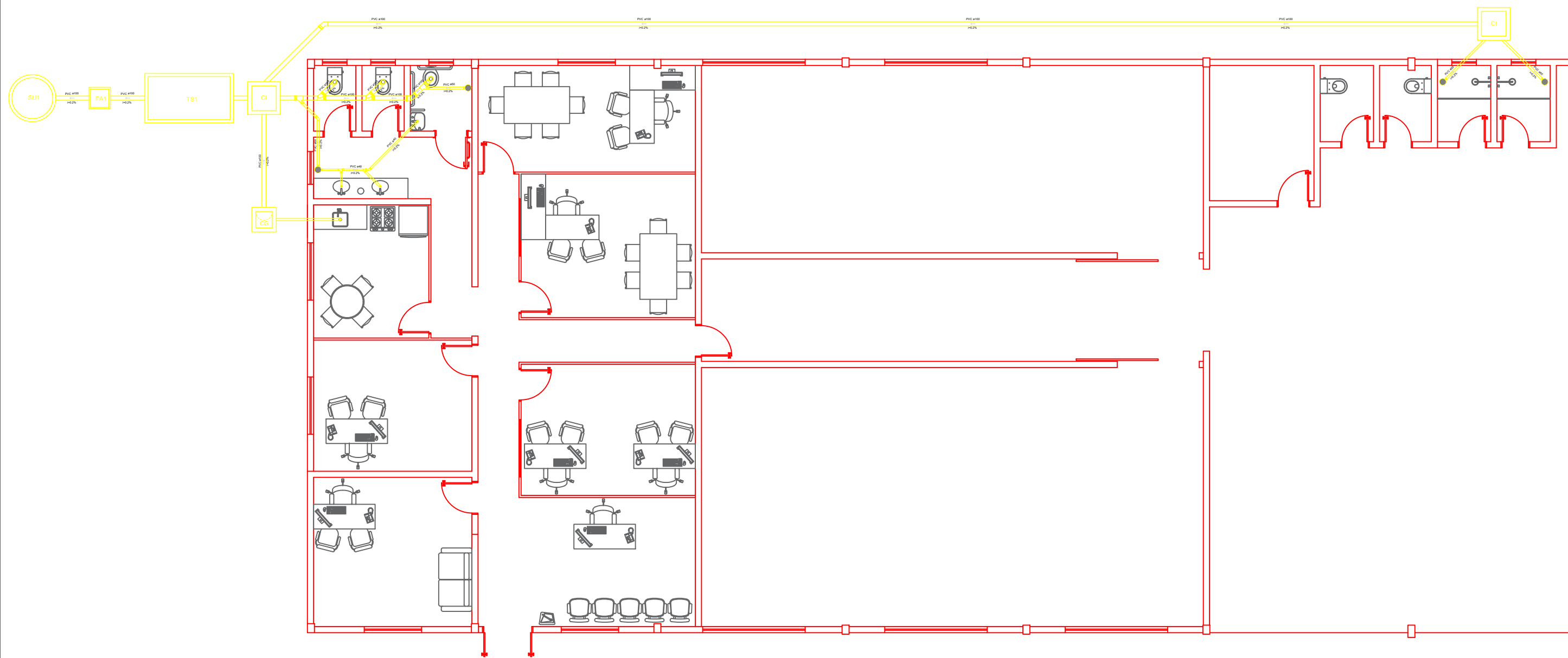
PROJETO HIDROSSANITÁRIO ESCALA 1:100
