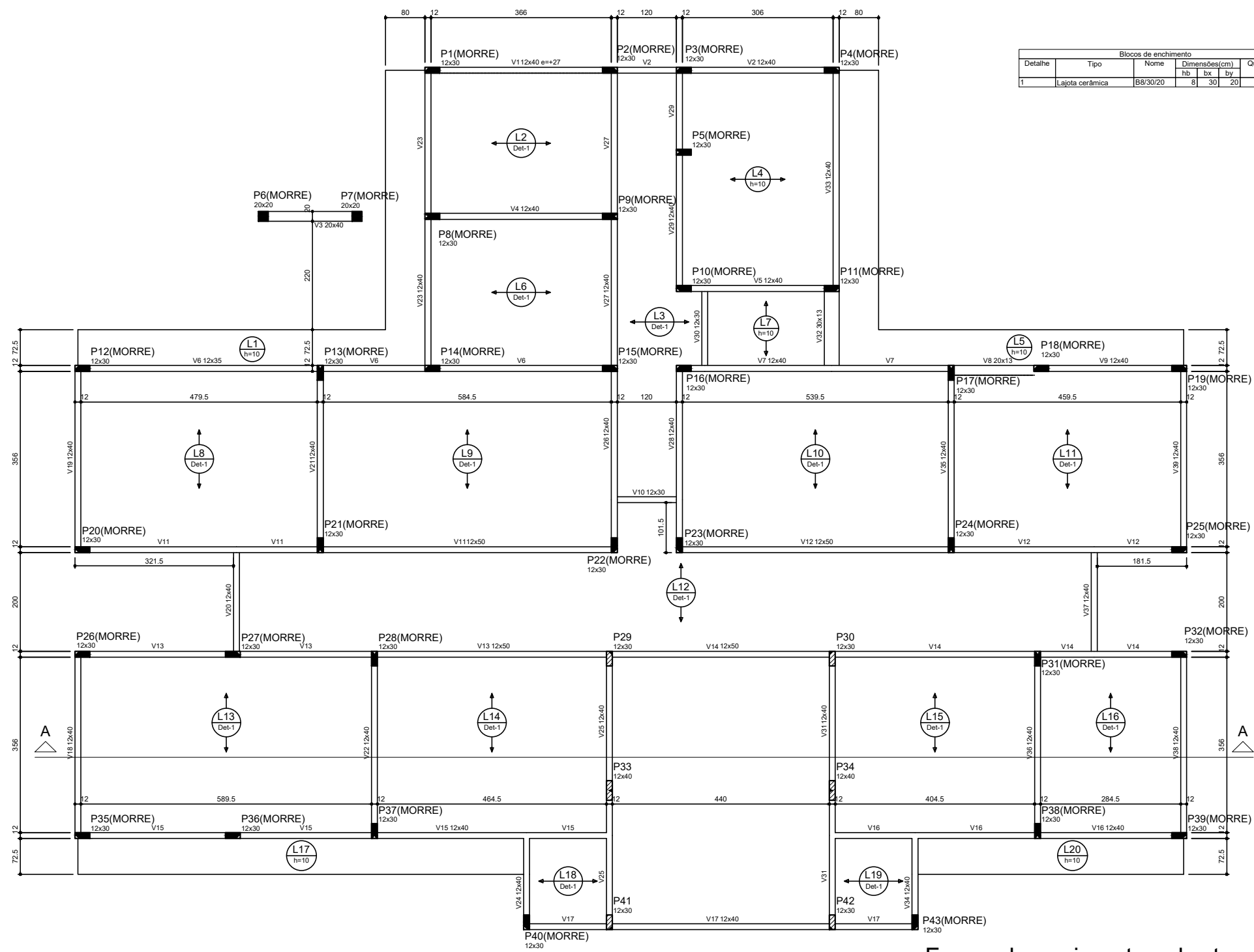
Forma do pavimento cobertura escala 1:50
